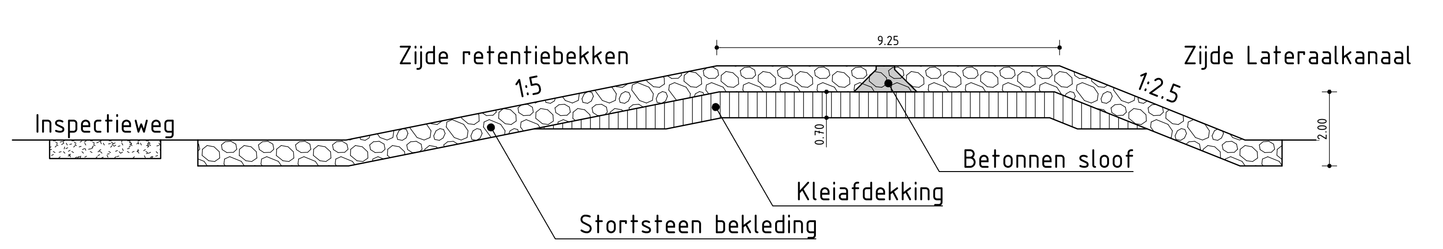
Technisch principeprofiel t.p.v. inlaat retentiebekken
