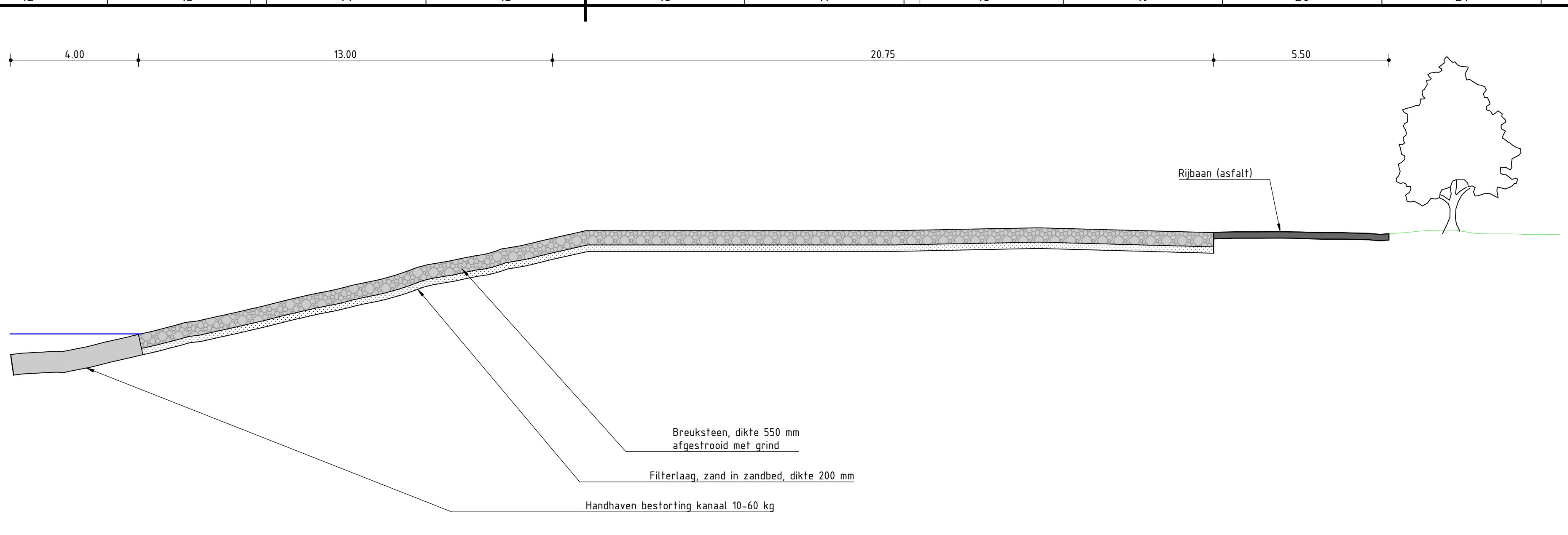
Technisch principeprofiel t.p.v. damverlaging
