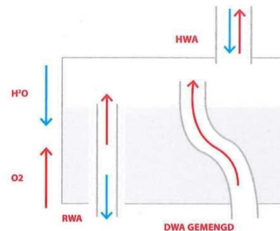
GEMENGD RIOOL
