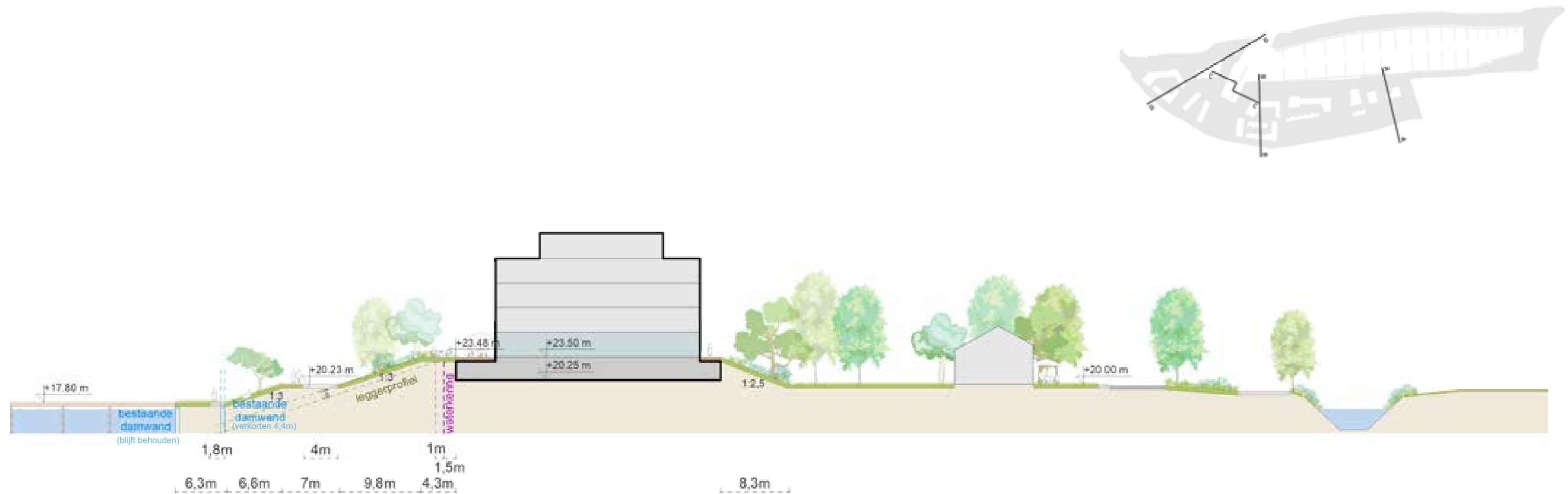
Principeprofiel A-A
