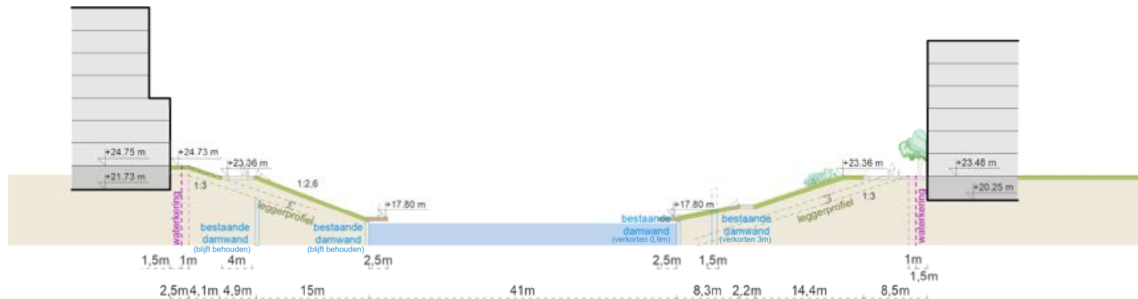
Principeprofiel C-C
